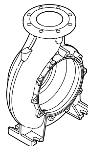
Рис. 15 Корпус насоса NB и NK с выпускным отверстием по оси
