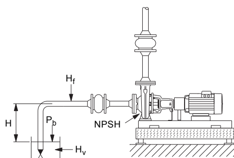
Рис. 37 Высота всасывания воды при положительном значении H
