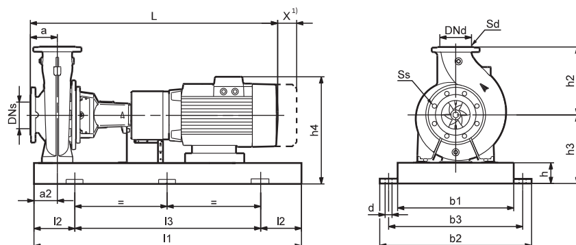
Рама основания EN/ISO, радиальный отвод
