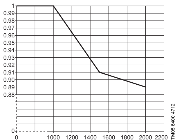
Рис. 31 Максимальная мощность двигателя в зависимости от высоты над уровнем моря
