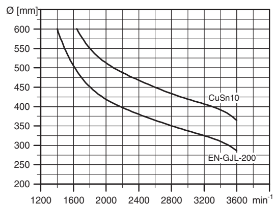
Рис. 52 Максимально допустимая частота вращения
