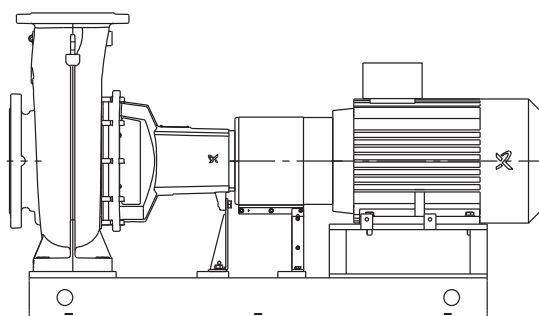
Рис. 62 Насос NK с С-образной плитой-основанием
