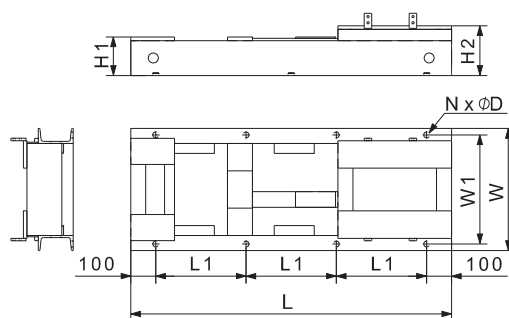
Рис. 65 С-образная рама-основание с 8 установочными отверстиями
