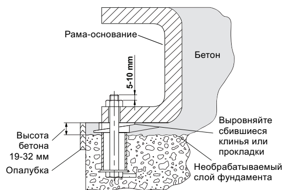
Рис. 44 Вид в разрезе фундамента с фундаментным болтом, бетонной заливкой и плитой-основанием
