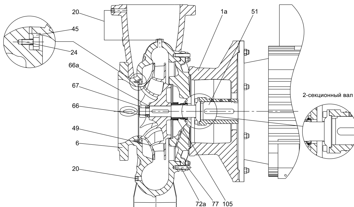
Рис. 7 Насос в разрезе (тангенциальный отвод), DN 200 и DN 250
