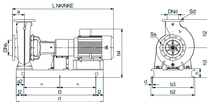
Рис. 66 Насос NK с С-образной плитой-основанием
