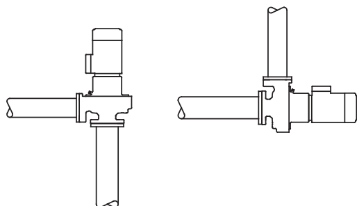
Рис. 47 Прямое соединение насоса с трубопроводом
