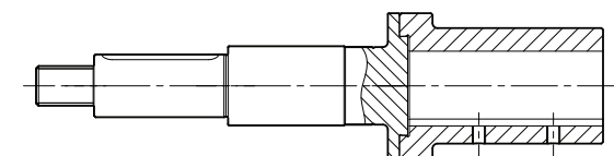
Рис. 21 2-секционный короткий вал, насос NB
