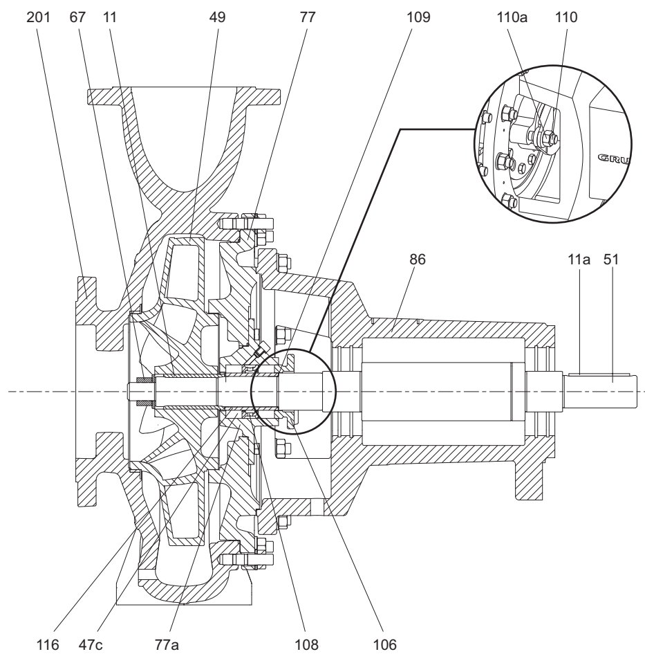
Рис. 10 Чертеж в разрезе, сальник
