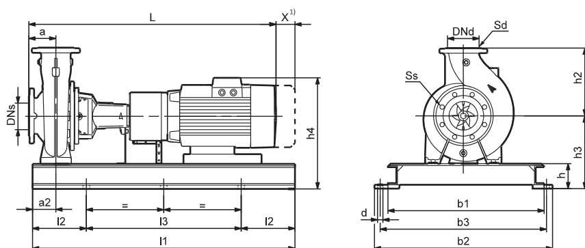
С-образная рама основания, радиальный отвод
