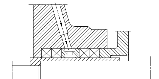
Рис. 17 Неохлаждаемый сальник типа SNE(x) с внутренней затворной жидкостью для перекачивания чистых жидкостей при всасывании или при давлении на входе до 4 бар
