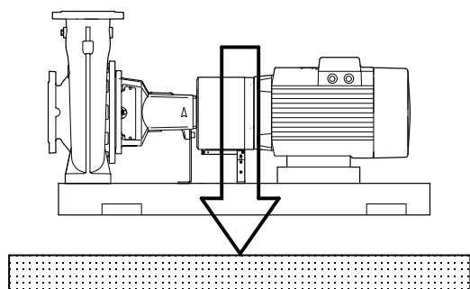
Рис. 40 Правильный фундамент
