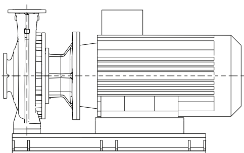
Рис. 67 Насос NB на плите-основании
