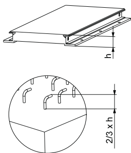
Рис. 43 Усиливающие стальные стержни, устанавливаемые в фундамент
