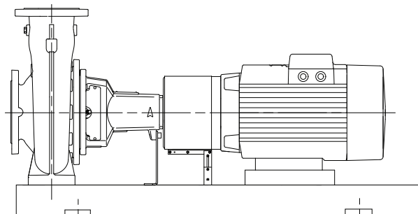
Рис. 61 Насос NK на плите-основании
