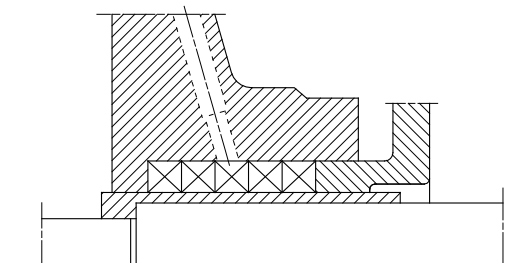
Рис. 18 Неохлаждаемый сальник типа SNO(x) без внутренней затворной жидкости для перекачивания чистых жидкостей при всасывании или при давлении на входе больше 4 бар
