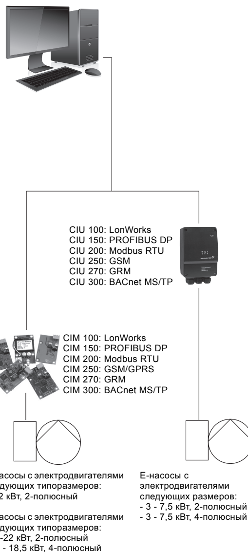
Рис. 58 Структура системы управления внутридомовыми коммуникациями
