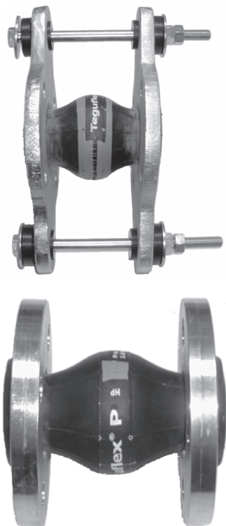
Рис. 49 Резиновые компенсаторы с ограничителями и без
