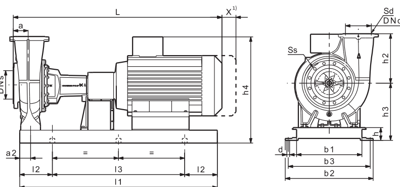
С-образная рама основания, тангенциальный отвод
