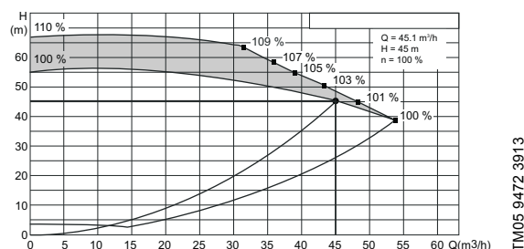
Рис. 51 Расширенный диапазон производительности Е-насосов
