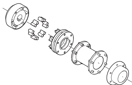
Рис. 23 Разъемная муфта (проставка)
