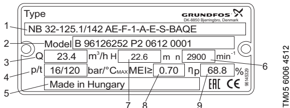
Рис. 5 Пример фирменной таблички
