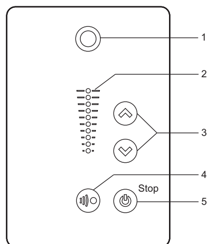
Рис. 55 Рабочая панель для 1,1 - 2,2 кВт 2-полюсных и 0,55 - 1,1 кВт 4-полюсных электродвигателей
