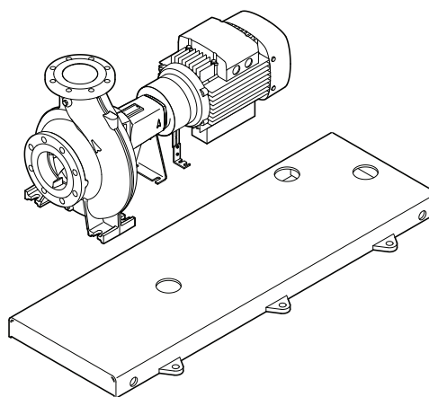
Рис. 42 Рама-основание, подготовленная для бетонирования
