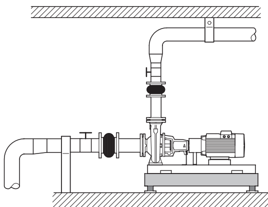
Рис. 46 Монтаж трубопровода
