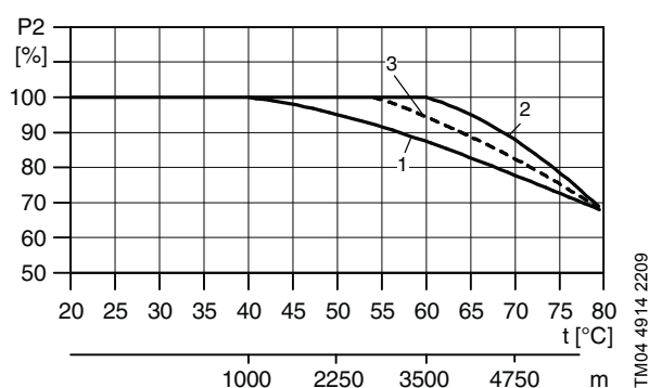
Рис. 30 Мощность двигателя в зависимости от температуры/высоты над уровнем моря
