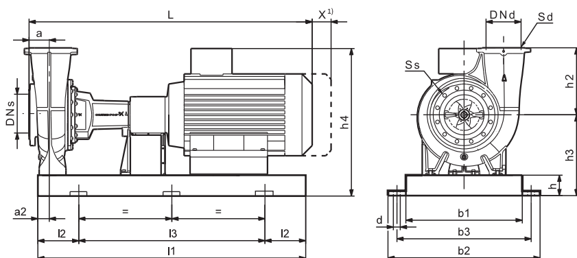
Рама основания EN/ISO, тангенциальный отвод
