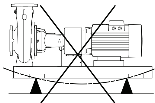
Рис. 41 Неправильный фундамент
