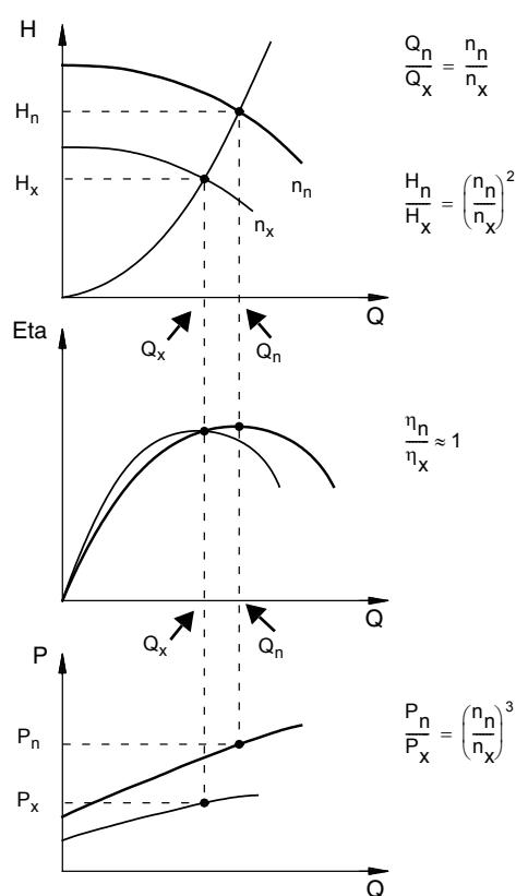
Рис. 54 Уравнения подобия
