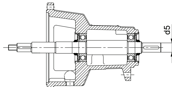
Рис. 16 Фонарь насоса и вал
