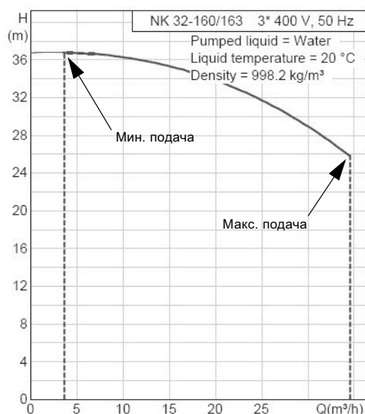
Рис. 32 На графике из Grundfos Product Center показан пример максимальной и минимальной допустимой подачи
