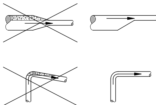
Рис. 45 Трубопроводы
