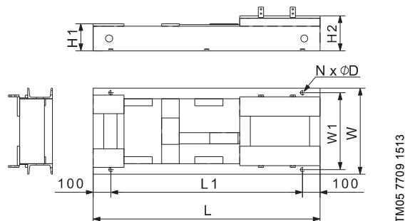
Рис. 63 С-образная рама-основание с 4 установочными отверстиями
