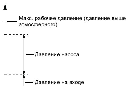
Рис. 35 Давление в насосе
