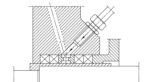
Рис. 19 Неохлаждаемый сальник типа SNF(x) с внешней затворной жидкостью для перекачивания загрязненных жидкостей и жидкостей с неприятным запахом
