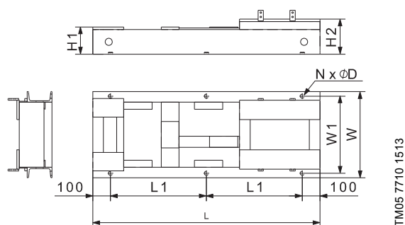
Рис. 64 С-образная рама-основание с 6 установочными отверстиями
