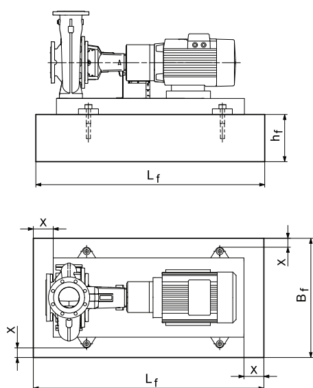
Рис. 39 Фундамент, X = мин. 100 мм
