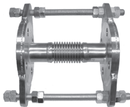
Рис. 50 Металлический компенсатор с ограничительными стержнями
