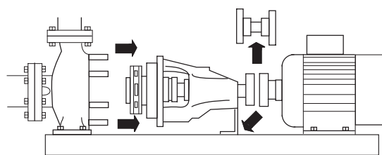
Рис. 4 Конструкция NK со съемной задней частью
